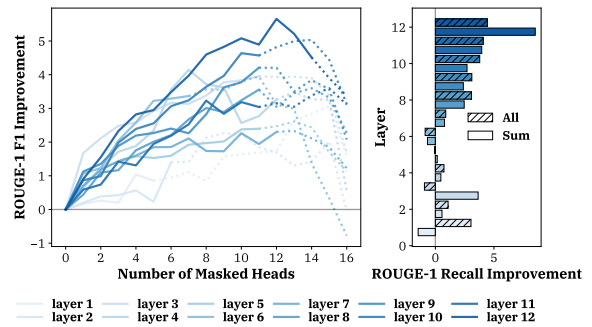
(b) NYT
