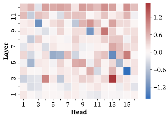
(b) NYT
