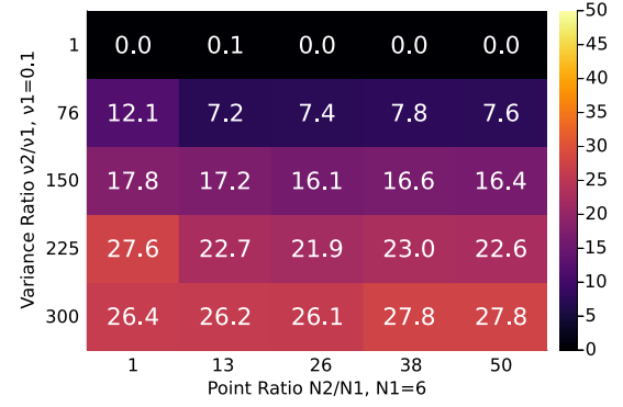
(d) ALPCAUS ( B=128 ) mean clustering error.
