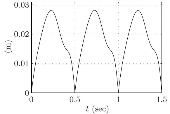
(d) p_2^y versus time.
